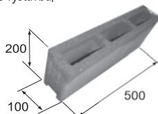
Priečková Murovacíá betónová tvárnica 10 D+D perodrážka MBT 10 D+D
