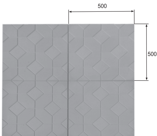
Záhradná dlažba Step 50
