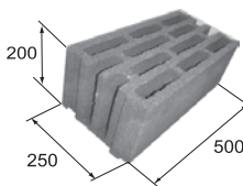
Obvodová nosná Murovacíá betónová tvárnica 25 P+D perodrážka MBT 25 P+D
